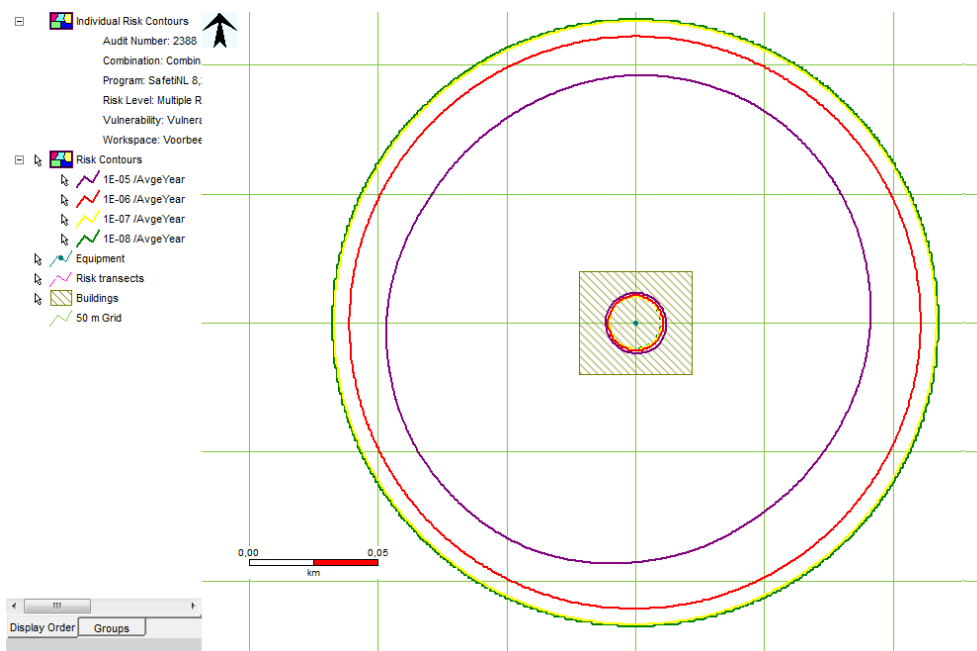
Figuur 9 Plaatsgebonden risicocontouren
