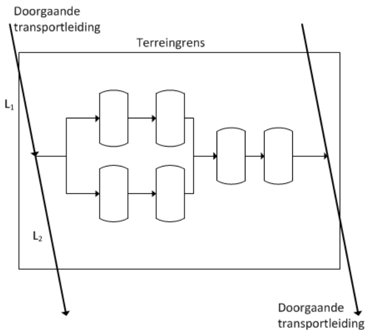
Figuur 20 Voorbeeld van een inrichting verbonden met doorgaande transportleidingen
