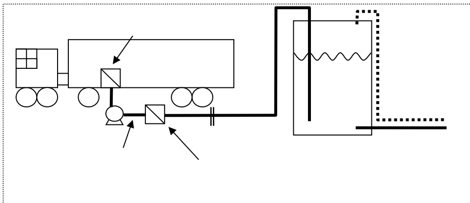
Figuur 7 Systeem afbakening propaan.
