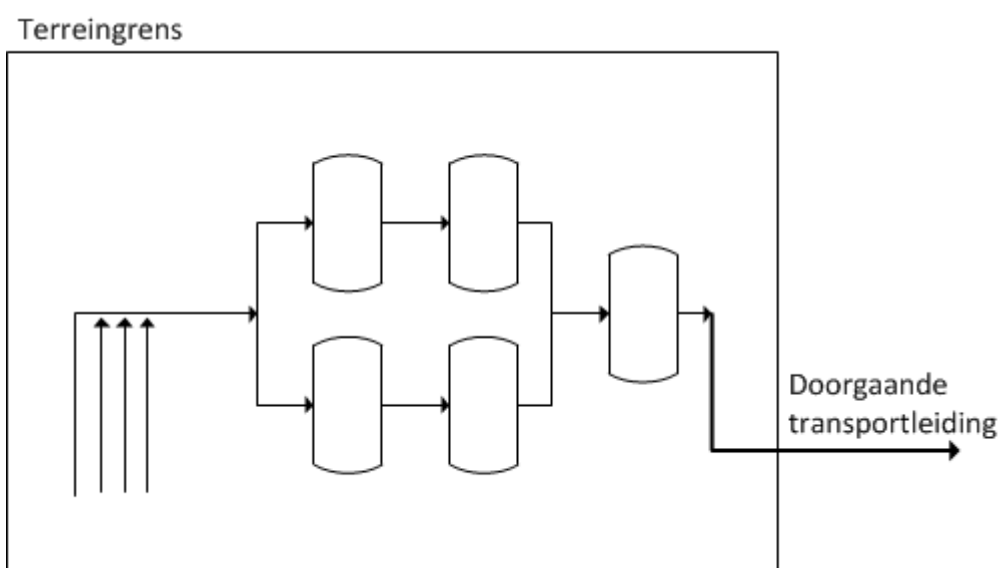
Figuur 22 Voorbeeld van een productielocatie
