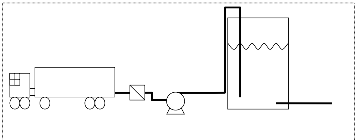
Figuur 6 Systeem afbakening ammoniak
