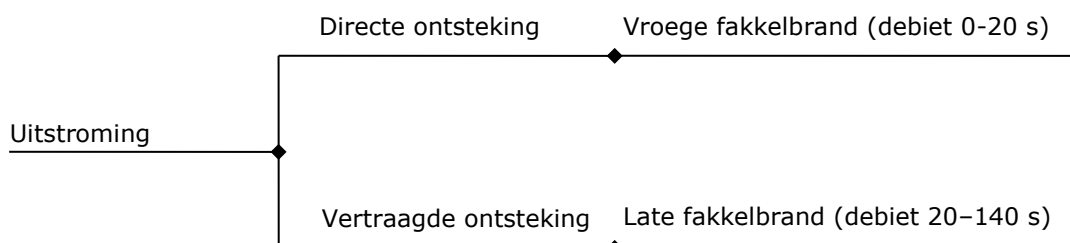
Figuur 16 Gebeurtenissenboom voor hogedruk gassystemen met een uitstroomduur groter of gelijk aan 20 s
