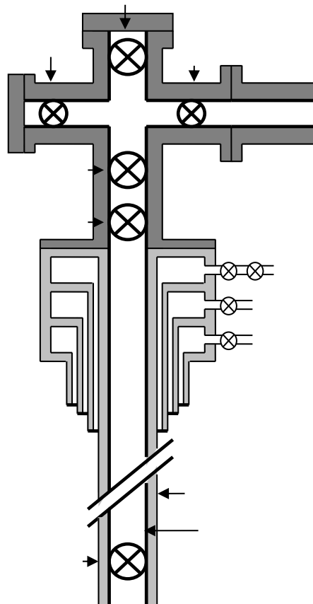
Figuur 15 Weergave van de put (inclusief 'christmas tree')
