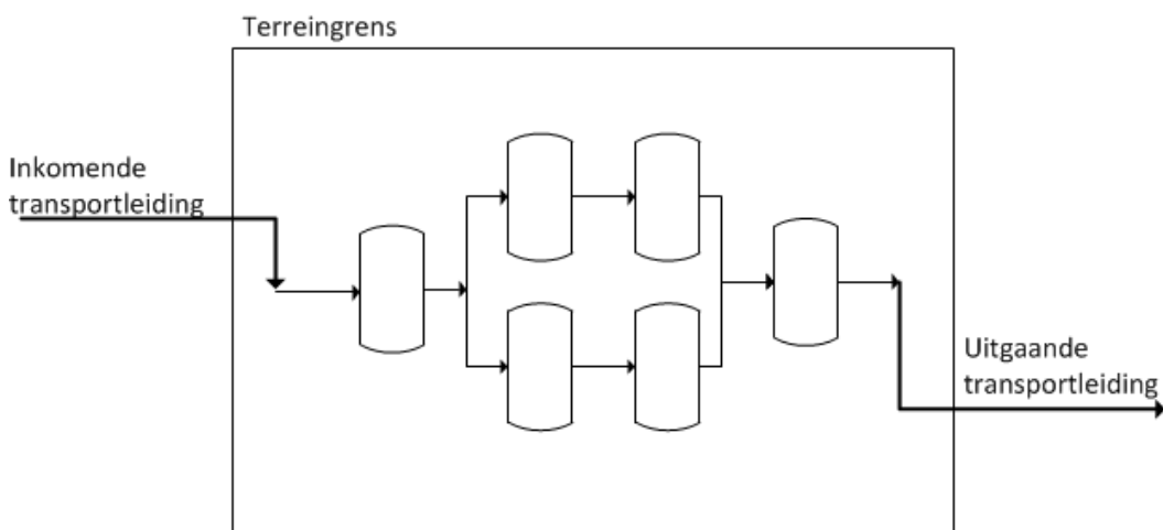
Figuur 18 Voorbeeld van een inrichting verbonden met één inkomende en één uitgaande transportleiding
