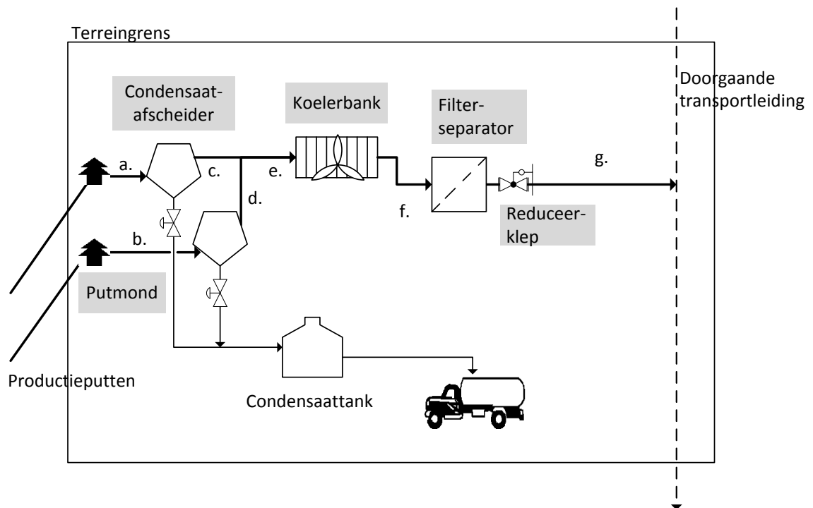
Figuur 23 Layout van de inrichting van het rekenvoorbeeld
