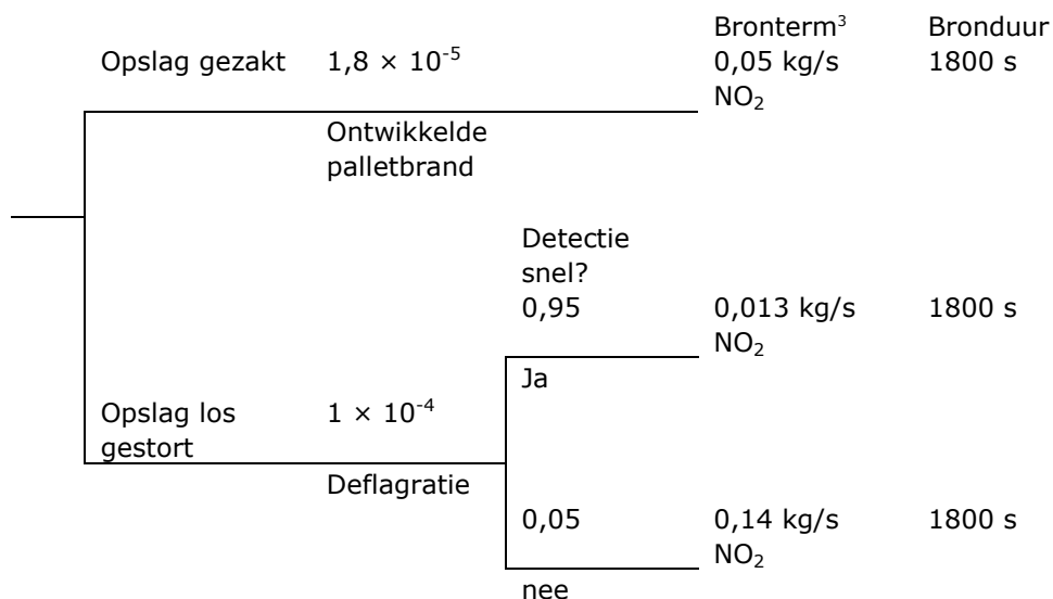
Figuur 2 Gebeurtenissenboom opslag meststoffen groep 2
