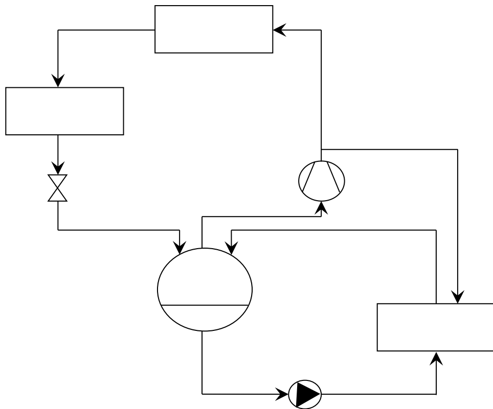
Figuur 3 Voorbeeld van een basisschema koelinstallatie
